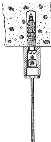
Anschrauben mit Dübel Seil mit ASS Klemmring
